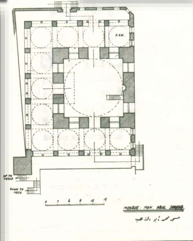
(شكل ١٠٧) مسقط أفق لمسجد محمد بك أبو الذهب بالأزهر
